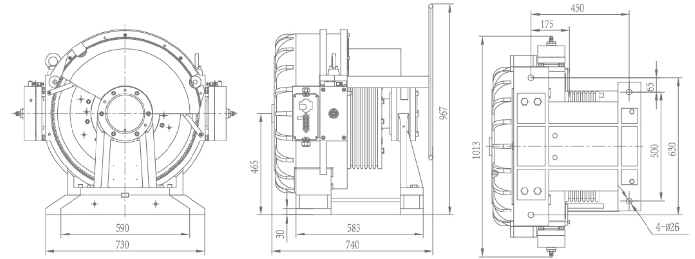
外观尺寸图 | Outline drawing
