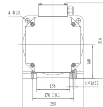
外观尺寸图 Outline drawing
