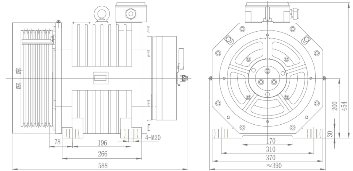
外观尺寸图 | Outline drawing
