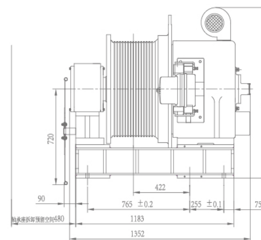
外观尺寸图 | Outline drawing
