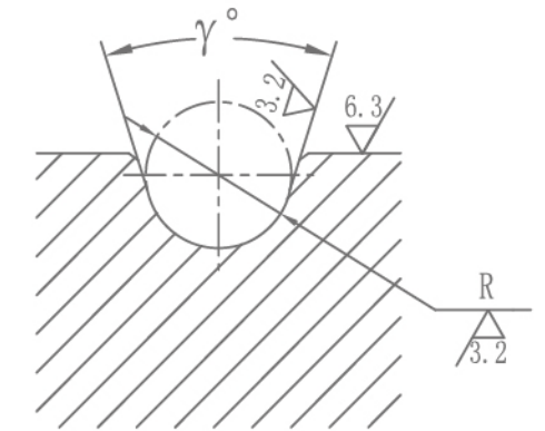
复绕槽型 (Double groove)
