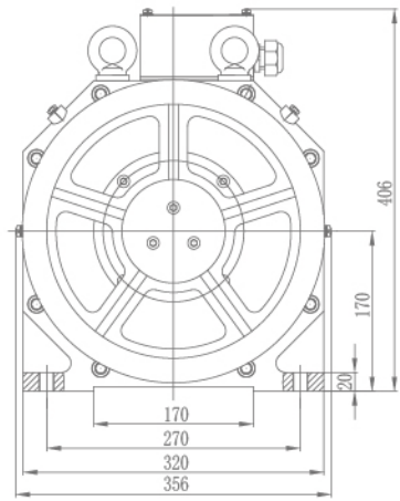
外观尺寸图 | Outline drawing
